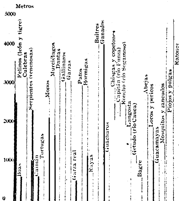
Diagrama representativo del escalonamiento de algunos animales en los Andes.
