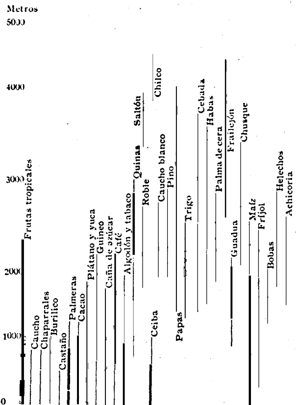
Diagrama representativo del escalonamiento de los principales vegetales en los Andes
