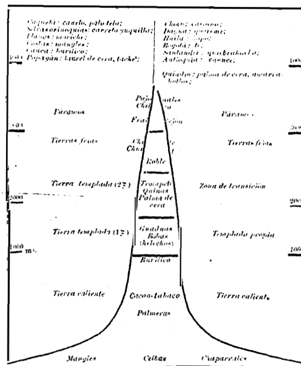
Diagrama del escalonamiento altimétrico de la flora colombiana
