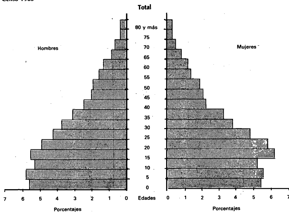
Gráfico 2 Quindío. Pirámide de población para el total, cabecera y resto. Censo 1985 a
