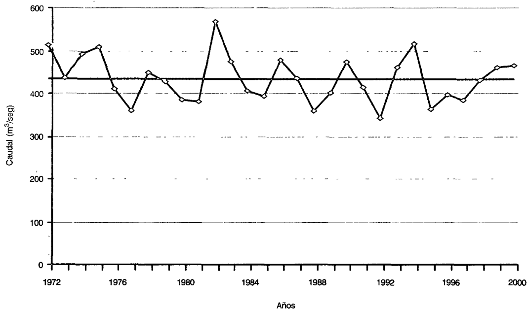
GRÁFICO 12.14 VARIACIÓN MULTIANUAL DE CAUDAL MEDIO DEL RÍO META 1972 - 2000 12.14.1 Estación Puente Lleras
