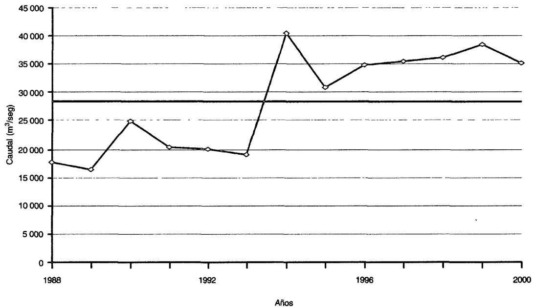
GRÁFICO 12.16 VARIACIÓN MULTIANUAL DE CAUDAL MEDIO DEL RÍO AMAZONAS 1988 - 2000 12.16.1 Estación Nazareth
