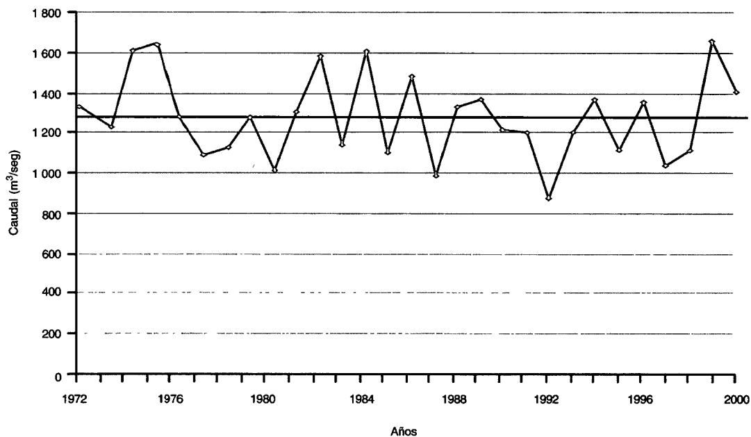
GRÁFICO 12.9 VARIACIÓN MULTIANUAL DE CAUDAL MEDIO DEL RÍO MAGDALENA 1972 - 2000 12.9.1 Estación Arrancaplumas
