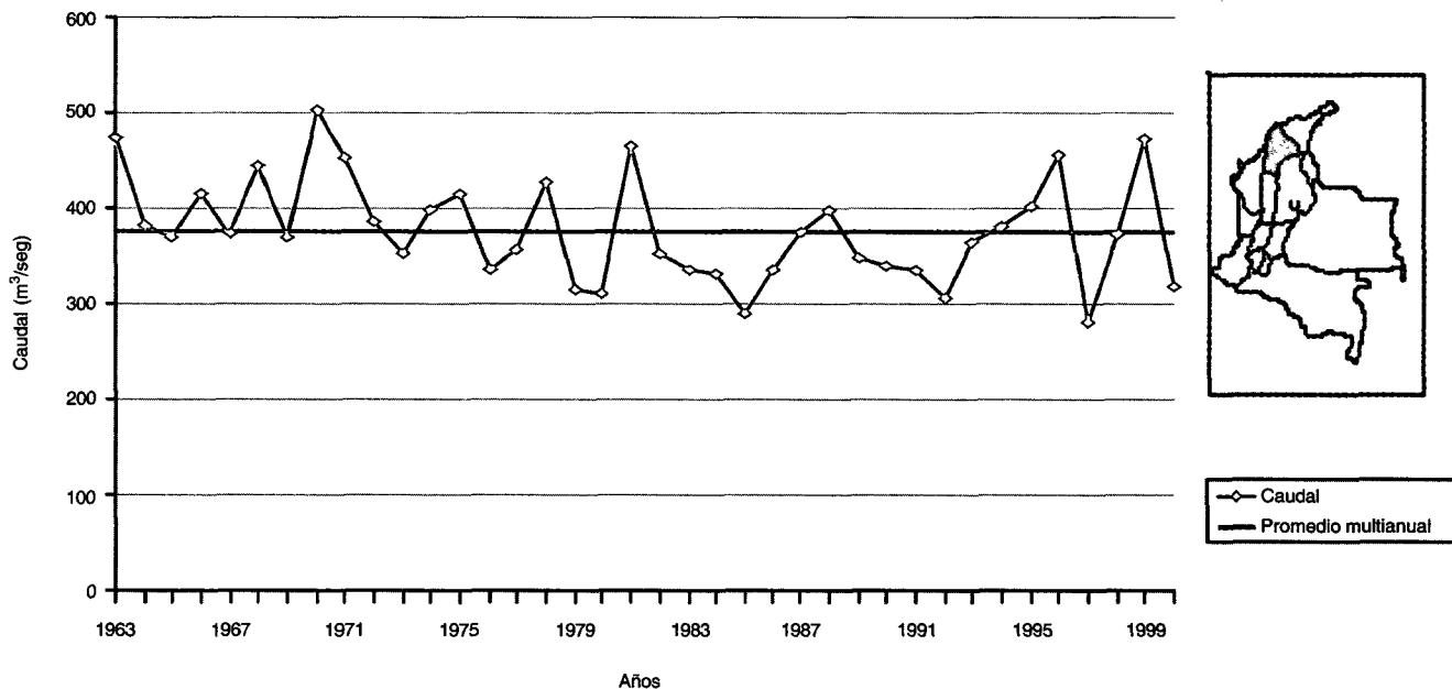
GRÁFICO 12.11 VARIACIÓN MULTIANUAL DE CAUDAL MEDIO DEL RÍO SINÚ 1963 - 2000 12.11.1 Estación Montería
