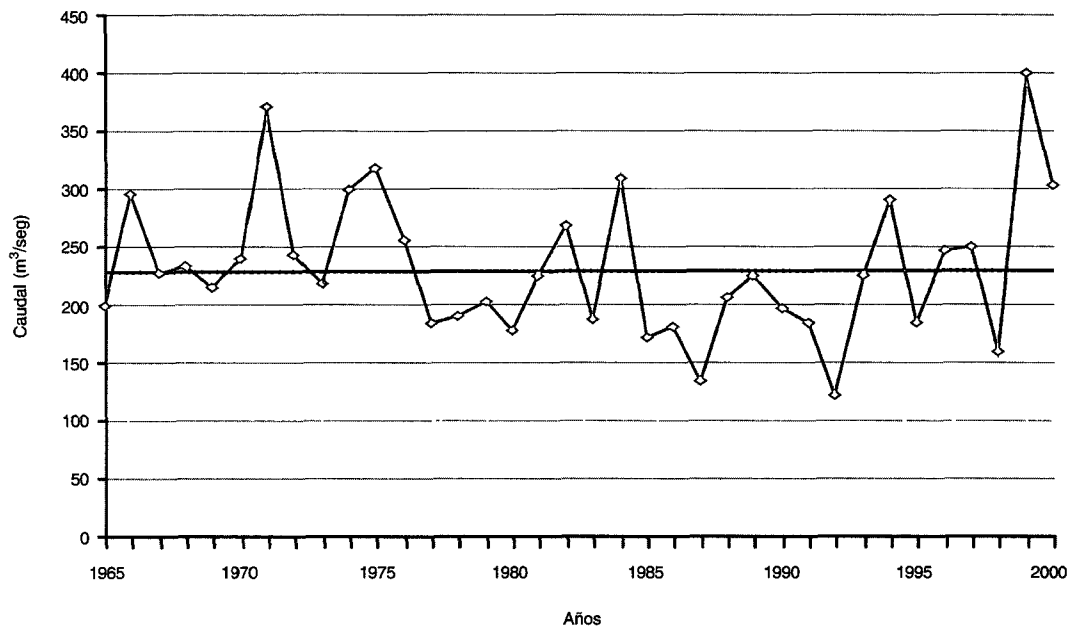
GRÁFICO 12.15 VARIACIÓN MULTIANUAL DE CAUDAL MEDIO DEL RÍO PATÍA 1965 - 2000 12.15.1 Estación Puente Guascas
