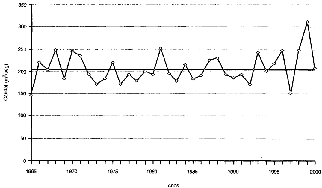
GRÁFICO 12.12 VARIACIÓN MULTIANUAL DE CAUDAL MEDIO DEL RÍO SAN JORGE 1965 - 2000 12.12.1 Estación Montelíbano
