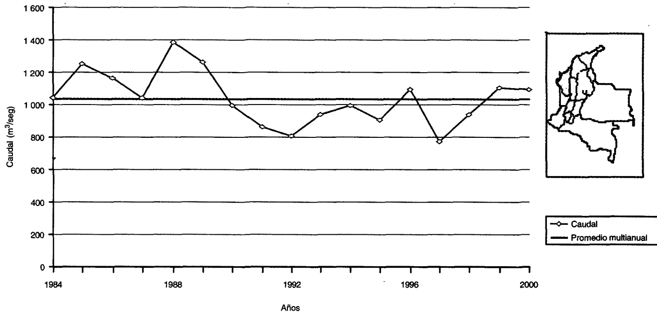
GRÁFICO 12.13 VARIACIÓN MULTIANUAL DE CAUDAL MEDIO DEL RÍO ATRATO 1984 - 2000 12.13.1 Estación Quibdó
