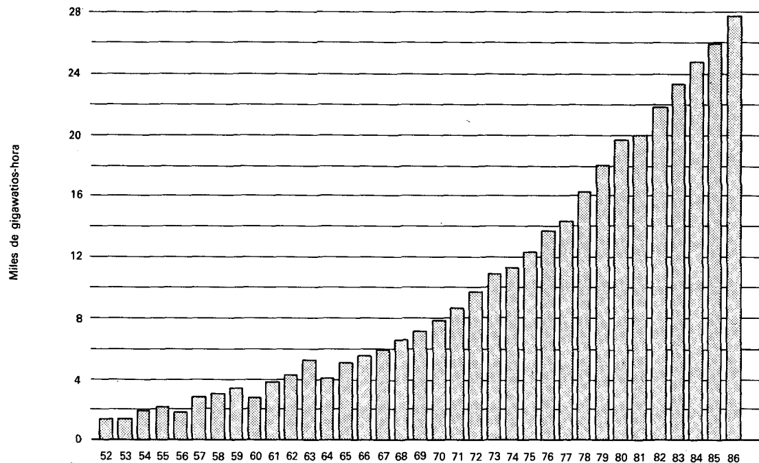
Gráfico 7.8 Energía eléctrica bruta generada Total país 1952-1986
