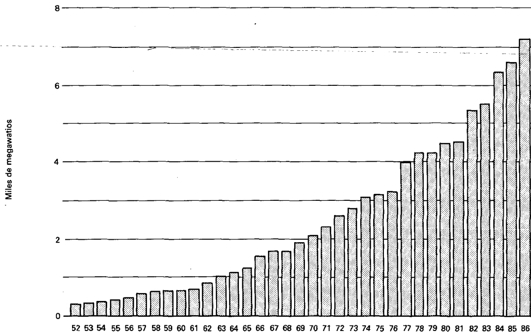
Gráfico 7.9 Capacidad eléctrica instalada Total nacional 1952-1986
