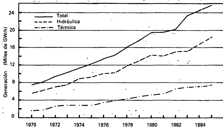
Gráfico 7.3.5 Generación eléctrica total y por origen 1970-1985
