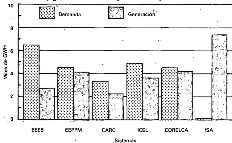
Gráfico 7.3.6 Demanda y generación de energía eléctrica por sistemas 1985
