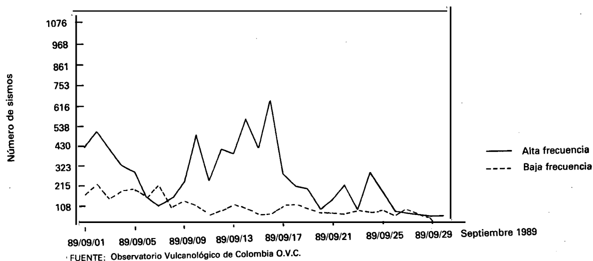
Gráfico 4 Sismos diarios en el Volcán Nevado del Ruiz
