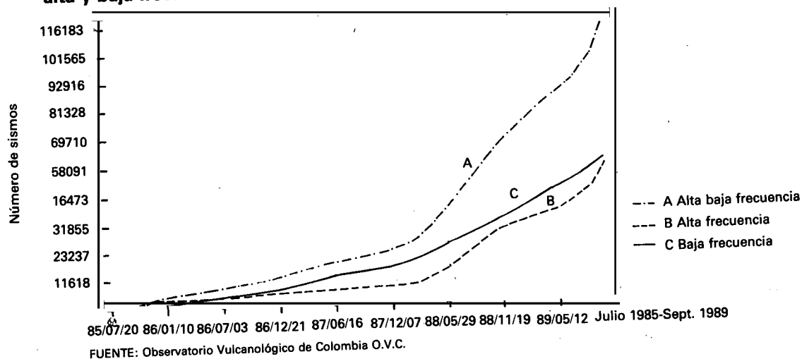
Gráfico 3 Sismos diarios acumulados Volcán Nevado del Ruiz alta y baja frecuencia
