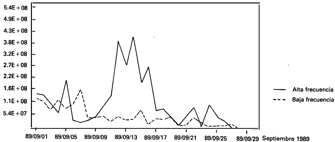
Gráfico 2 Energía liberada diaria alta y baja frecuencia en el Volcán Nevado del Ruiz
