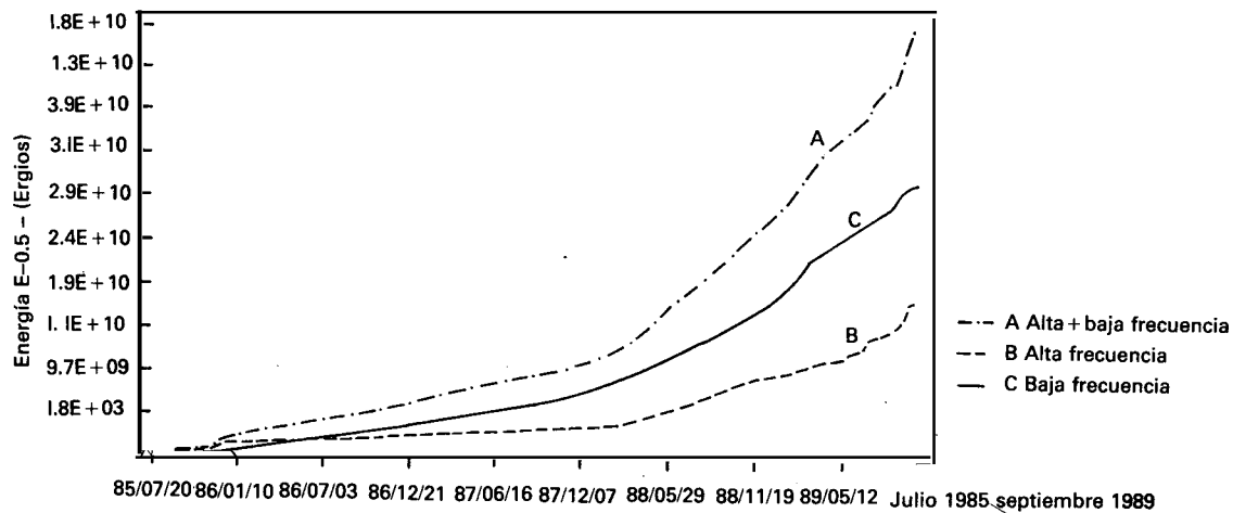
Gráfico 1 Energía acumulada liberada en el Volcán Nevado del Ruiz
