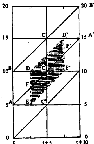
Gráfico 1 Diagrama de Lexis para el cálculo de K_{5-9} en un período intercensal de 10 años.
