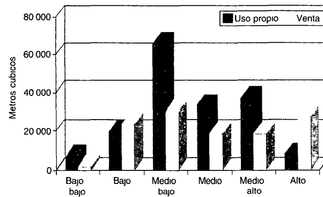
Grafico 13 Consumo de premezclado inicio obra, por estratos socioeconomicos, segun uso propio II trimestre de 2001
