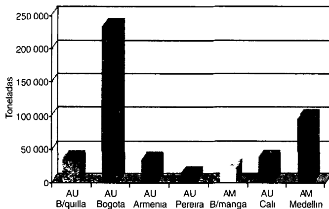
Grafico 4 Consumo total cemento inicio obras, por areas urbanas y metropolitanas II trimestre de 2001
