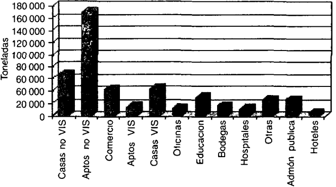
Grafico 2 Consumo total de cemento inicio obras, por destinos y tipo de edificacion (VIS no VIS) II trimestre de 2001
