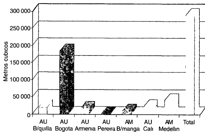
Grafico 16 Consumo de premezclado inicio obras, por areas urbanas y metropolitanas II trimestre de 2001
