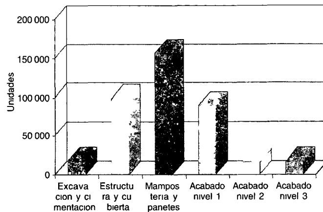
Grafico 22 Consumo total bloques de cemento mes obras, por capitulos constructivos II trimestre de 2001
