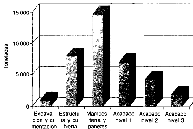
Grafico 10 Consumo total de cemento mes obras, por capitulos constructivos II trimestre de 2001
