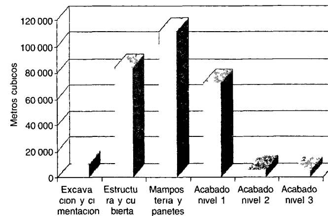
Grafico 14 Consumo total de premezclado inicio obras, por capitulos constructivos II trimestre de 2001
