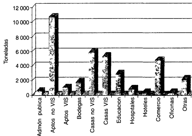
Grafico 10 Consumo total de cemento mes obras, por capitulos constructivos II trimestre de 2001
