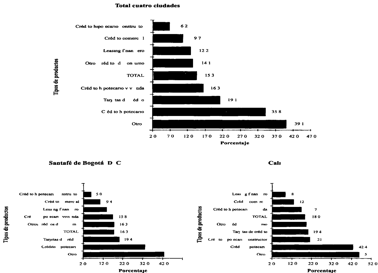
Gráfico 4 Participación porcentual de los problemas de recaudo en el total de las operaciones de cartera según tipos de productos y ciudades 1996
