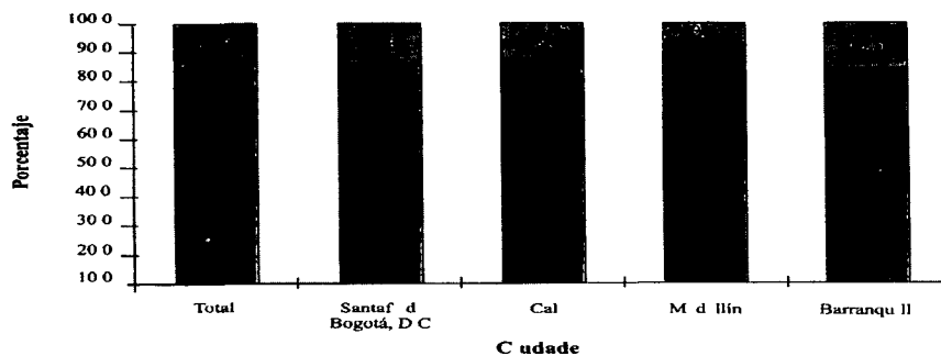
Gráfico 3 Participación porcentual de los problemas de cartera en el total de operaciones según ciudades 1996
