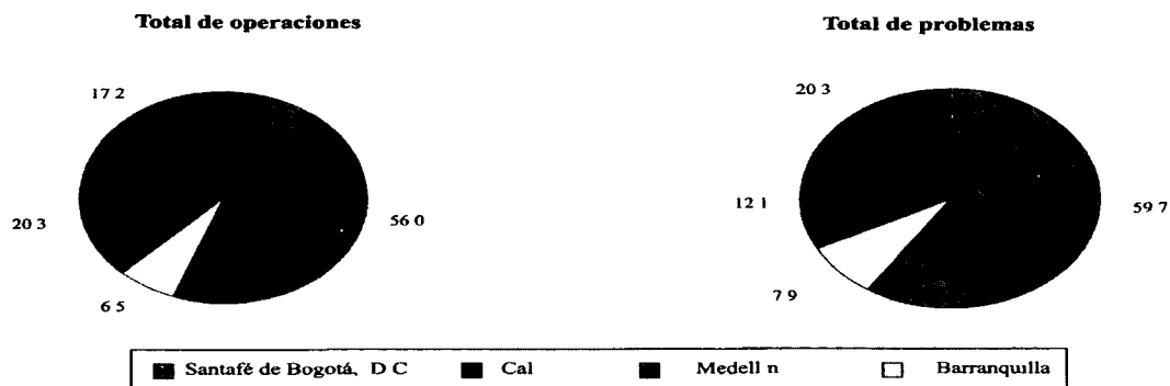
Gráfico 2 Distribución porcentual de las operaciones y los problemas de recaudo, por ciudades 1996
