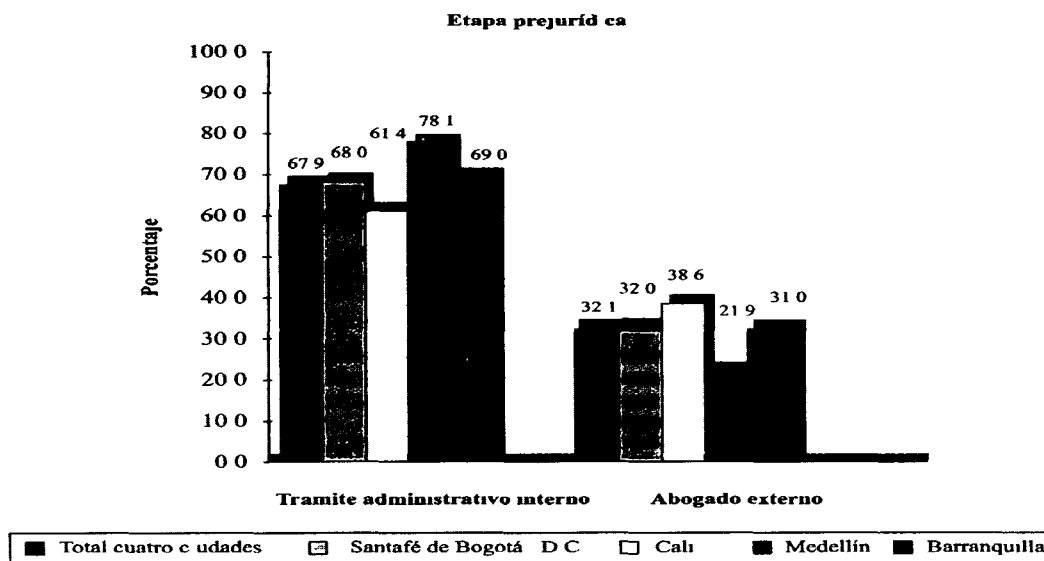
Gráfico 7 Participación porcentual de los problemas de cartera por ciudades y forma de solución según etapa del proceso 1996
