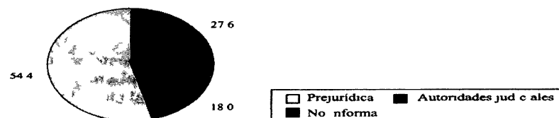
Gráfico 6 Distribución porcentual de los problemas de cartera, por tipos de solución según ciudades 1996
