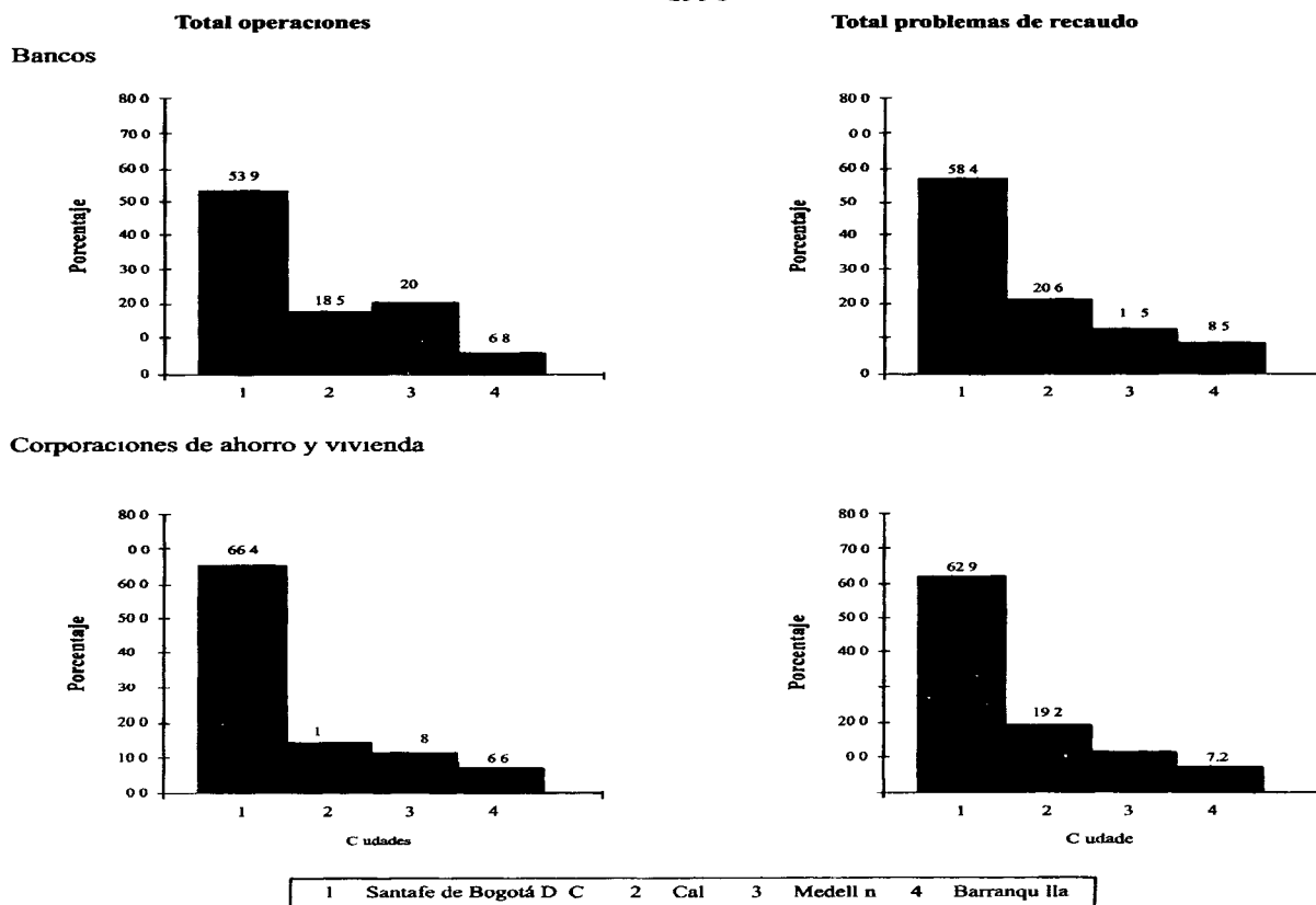
Gráfico 5 Distribución porcentual de las operaciones de cartera y los problemas de recaudo por entidades segun ciudades 1996
