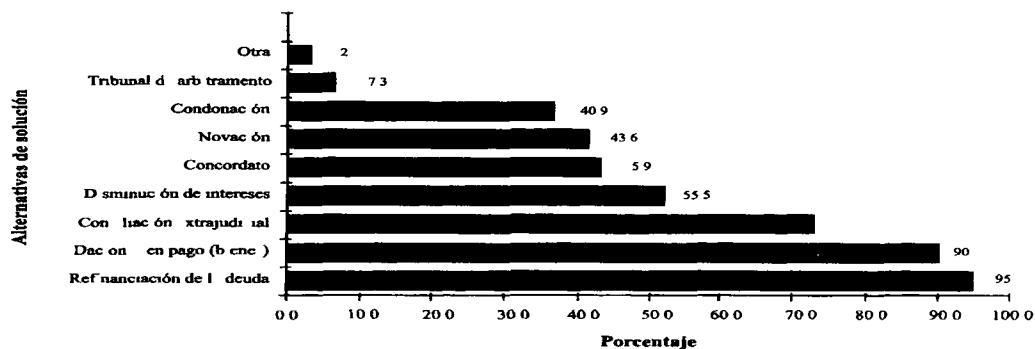
Gráfico 12 Participación de las alternativas de solución de las dificultades de cartera en el total de las entidades Total cuatro ciudades 1996
