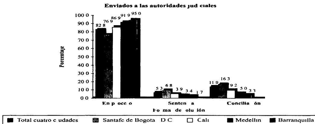
Gráfico 7 (conclusión) Participación porcentual de los problemas de cartera por ciudades y forma de solución según etapa del proceso 1996
