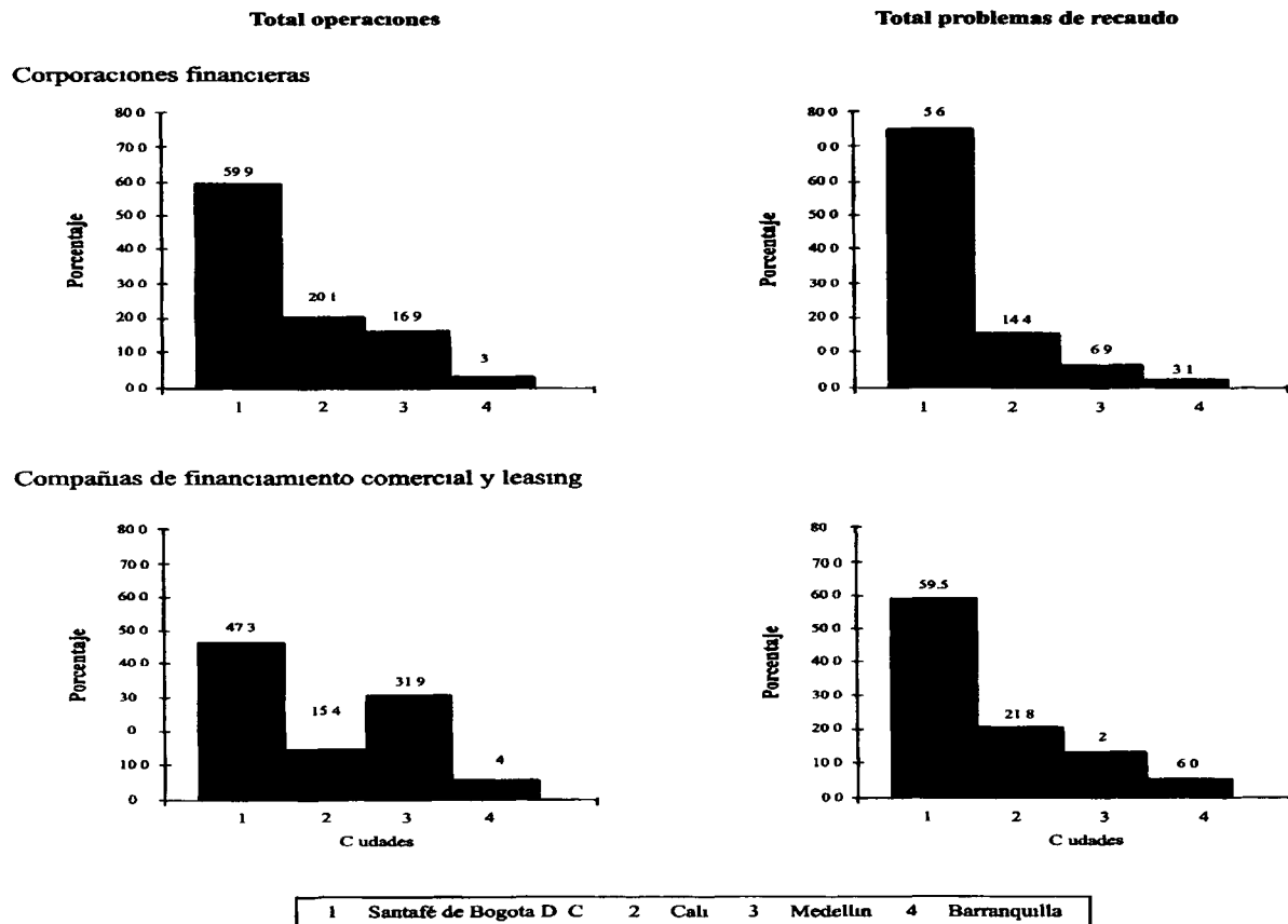
Gráfico 5 (conclusión) Distribución porcentual de las operaciones de cartera y los problemas de recaudo por entidades, según ciudades 1996
