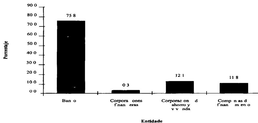
Gráfico 9 Distribución porcentual de los problemas de cartera enviados a las autoridades judiciales por entidades Total cuatro ciudades 1996
