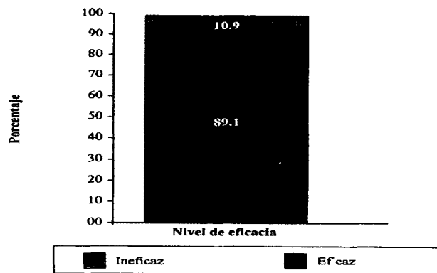
Gráfico 13 Distribución de la calificación sobre la gestión en las etapas prejurídicas por eficacia Total cuatro ciudades 1996
