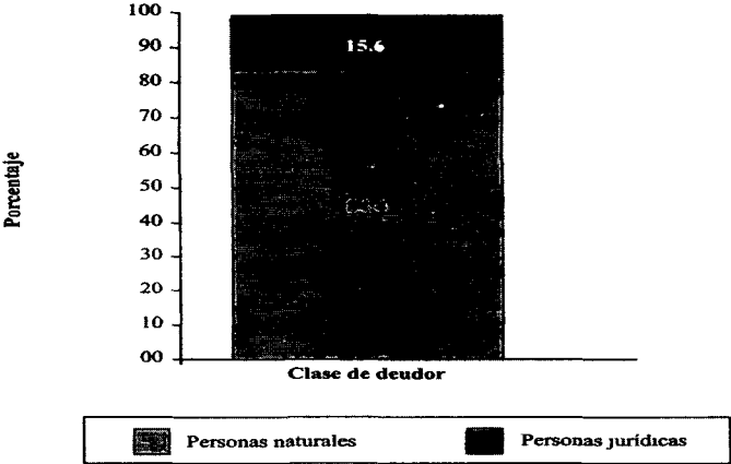
Gráfico 11 Distribución de los problemas de recaudo por clase de deudor Total cuatro ciudades 1996
