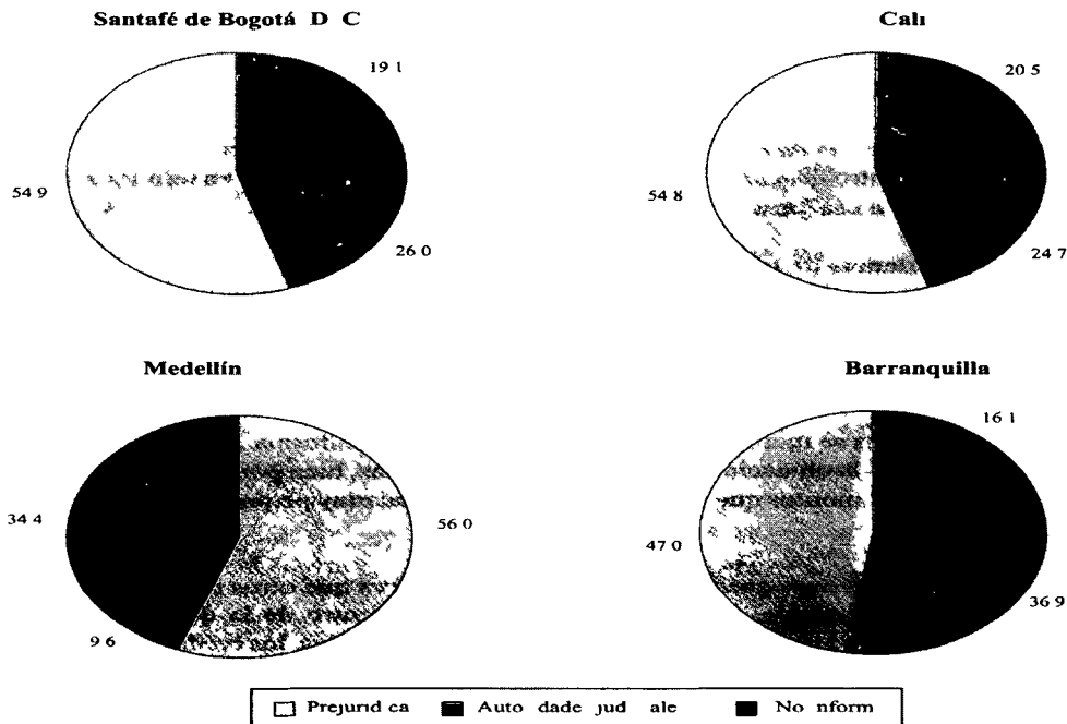
Gráfico 6 (conclusión) Distribución porcentual de los problemas de cartera por tipos de solución según ciudades 1996
