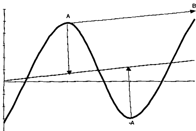
Gráfica 2 Función seno con tendencia
