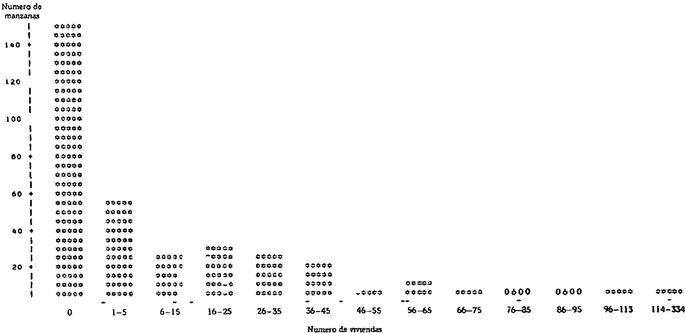
RECUESTO DE EDIFICACIONES Y VIVIENDAS MEDELLIN CABECERA 1981 Grafico 3 12 Diagrama de barras de la frecuencia de manzanas, segun el numero de viviendas Comunidad 35
