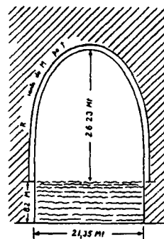
Corte de proyecto del tunel para el canal interoceánico Atrato Napipi proyectado por Fredrick C. H. en 1875
