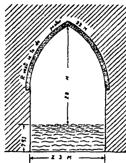
Corte de proyecto del tunel para el canal interoceánico Atrato Napipi proyectado por el Almirante Thomas Oliver Selfridge en 1873
