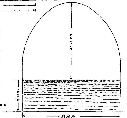
Corte de proyecto para el tunel Atrato Truando sin esclusas proyectado por Antoni L. Armentis en 1943 a una profundidad de 57 pies de calado
