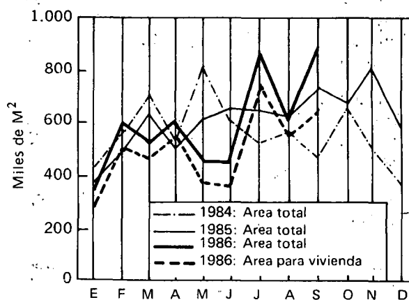
Gráfico 2 Área para construcción aprobada Total 11 áreas metropolitanas Enero 1984-septiembre 1986
