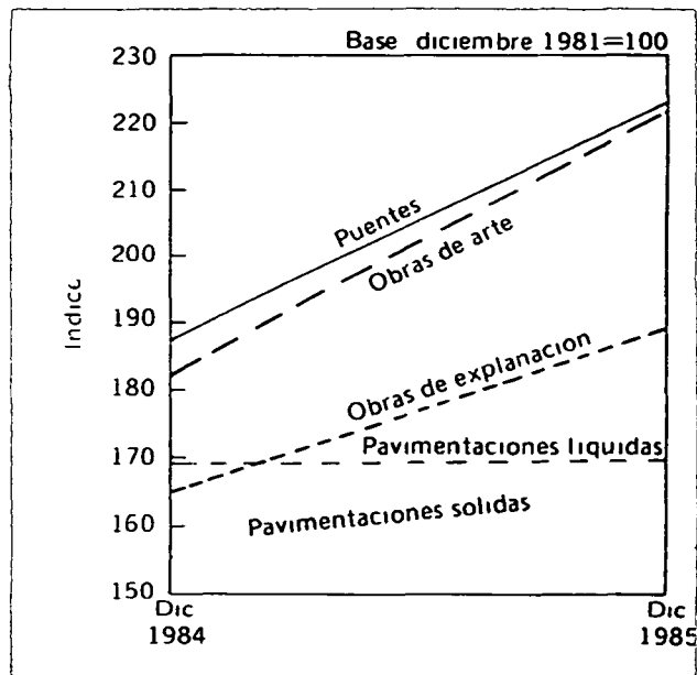
Grafico 2 Indice de costos de materiales para construccion pesada, por grupos de obras Diciembre 1984—diciembre 1985
